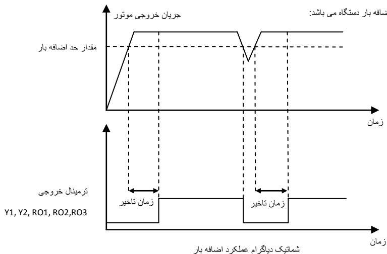
شماتیک دیگرام عملکرد اضافه بار
