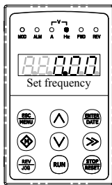
Fig.b Waiting status, display waiting status parameter
